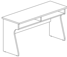
Training Desk (H400 modesty panel) R1T1205 W1200×D500×H750 R1T1405 W1200×D500×H750 R1T1506 W1500×D600×H750 R1T1606 W1200×D600×H750 R1T1806 W1800×D600×H750
