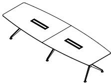
Model: MG-MM3012 3000W x 1200D x 750H Model: MG-MM3612 3600W x 1200D x 750H
