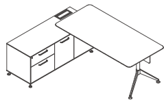
Model:MG-MLD1.2118 2150W x 1850Dx 750H
