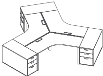
Y 型三人工作站 Workstation Three Persons Workstation-type Y M10-FY3-1006 3199×2770×H750 M10-FY3-1206 3545×3070×H750 M10-FY3-1406 3891×3370×H750
