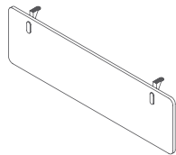
挡板 (MFC) Hanging Modesty Panel M10B-HMP-0935 900×T18×H350(配 1400 长台 /fit W1400 Desk) M10B-HMP-1135 1100×T18×H350(配 1600 长台 /fit W1600 Desk) M10B-HMP-1335 1300×T18×H350(配 1800 长台 /fit W1800 Desk) M10B-HMP-1635 1600×T18×H350(配 2100 长台 /fit W2100 Desk)
