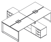
D 型四人工作站 Four Persons Workstation-type D M10-MD4-1407 2800×2800×H750 M10-MD4-1507 3000×2800×H750 M10-MD4-1608 3200×2800×H750
