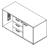
活动柜 Mobile Side Pedestal M10-SC01-1205 1200×500×H600
