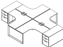
X 型四人工作站 Four Persons Workstation-type X M10-MX4-1407 3800×2800×H750 M10-MX4-1507 4000×3000×H750 M10-MX4-1608 4200×3200×H750
