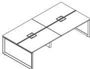
B 型四人工作站 Four Persons Workstation-type B M10-MB4-1206 2400×1200×H750 M10-MB4-1407 2800×1400×H750 M10-MB4-1507 3000×1400×H750 M10-MB4-1608 3200×1600×H750
