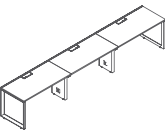
A 型三人工作站 Three Persons Workstation-type A M10-MA3-1206 3600×600×H750 M10-MA3-1407 4200×700×H750 M10-MA3-1507 4500×700×H750 M10-MA3-1608 4800×800×H750
