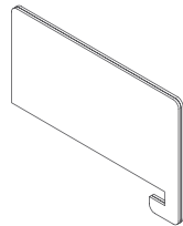
侧桌屏 (吸音板) Side Screen--Acoustic Panel ZF-PET-D060 550×T18×H370(配 600 宽台 /fit D600 Desk) ZF-PET-D070 650×T18×H370(配 700 宽台 /fit D700 Desk) ZF-PET-D080 750×T18×H370(配 800 宽台 /fit D800 Desk)
