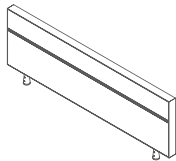
桌屏 (40 屏风) Desk Mounted Screen ZF-F40-W08 800×T40×H350(配 1200 长台 /fit W1200 Desk) ZF-F40-W10 1000×T40×H350(配 1400 长台 /fit W1400 Desk) ZF-F40-W11 1100×T40×H350(配 1500 长台 /fit W1500 Desk) ZF-F40-W12 1200×T40×H350(配 1600 长台 /fit W1600 Desk)
