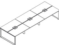
B 型六人工作站 Six Persons Workstation-type B M10-MB6-1206 3600×1200×H750 M10-MB6-1407 4200×1400×H750 M10-MB6-1507 4500×1400×H750 M10-MB6-1608 4800×1600×H750
