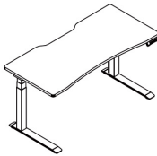
方形独立桌 Rectangular table HAT-MS1507 W1500*D700 HAT-MS1807 W1800*D700
